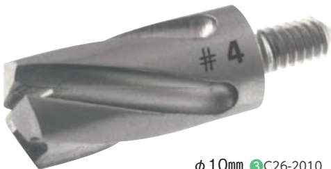
φ 10mm ③C26-2010 φ 12mm ④C26-2012 φ 14mm ⑤C26-2014
