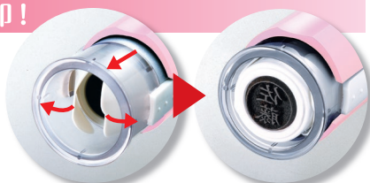
ウィングシャッター機構
