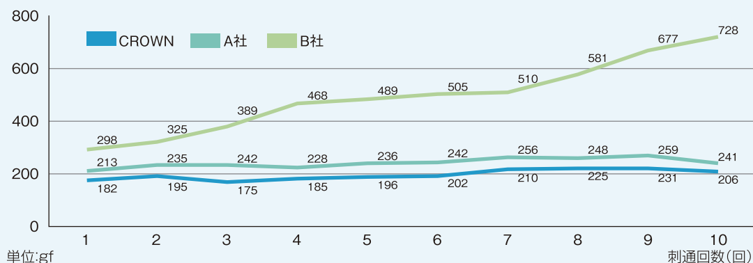
角針 刺通抵抗値 (13mm)
